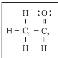
Acetaldehyde, \text{CH}_3\text{COH}
